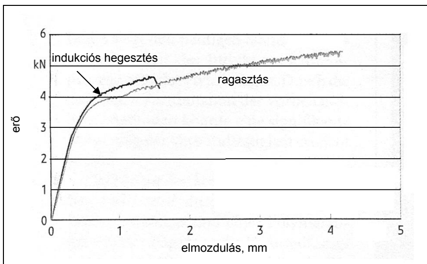
1. ábra Erő-elmozdulás diagram az indukciósan hegesztett, ill. ragasztott próbatesteken
